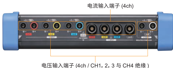
系列共通 侧面
