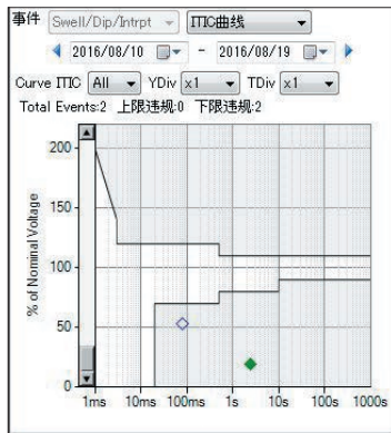
ITIC 曲线的界面示例
