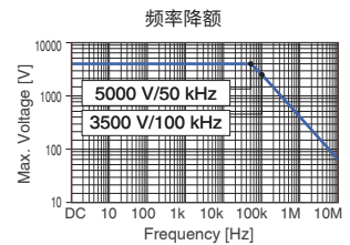
AC/DC 高压分压器VT1005
