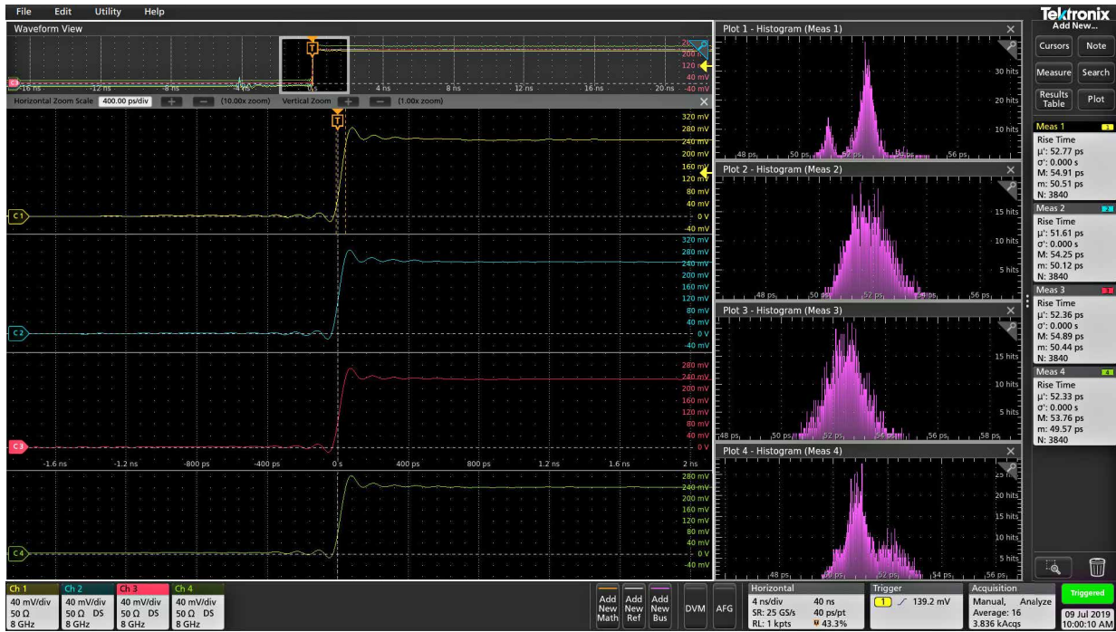
各输入上的高采样率可实现新的密度性能。在本例中，4 个通道以 25 GS/s 的速度测量上升边沿~52 ps。
