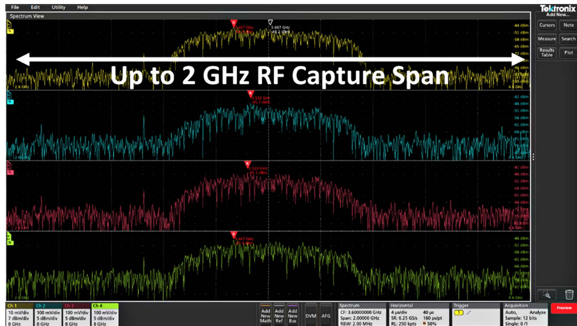
直观的频谱分析仪控制功能如中心频率、频宽和解析带宽 (RBW) 独立于时域控制功能，可以简便地进行设置，实现频域分析。频谱视图适用于每个模拟输入，支持多通道混合域分析。
